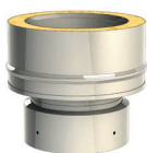
Adaptador flex a DW-ECO 1.0
